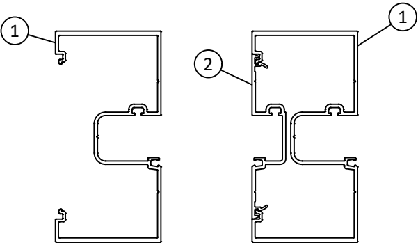
LIGHT JAMB - J1
