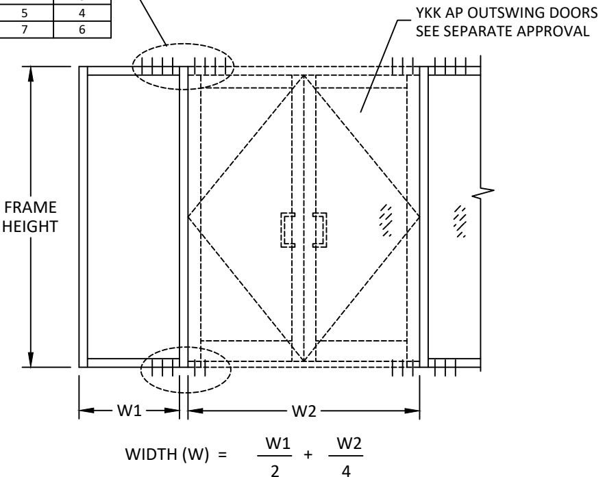
DOUBLE DOOR
